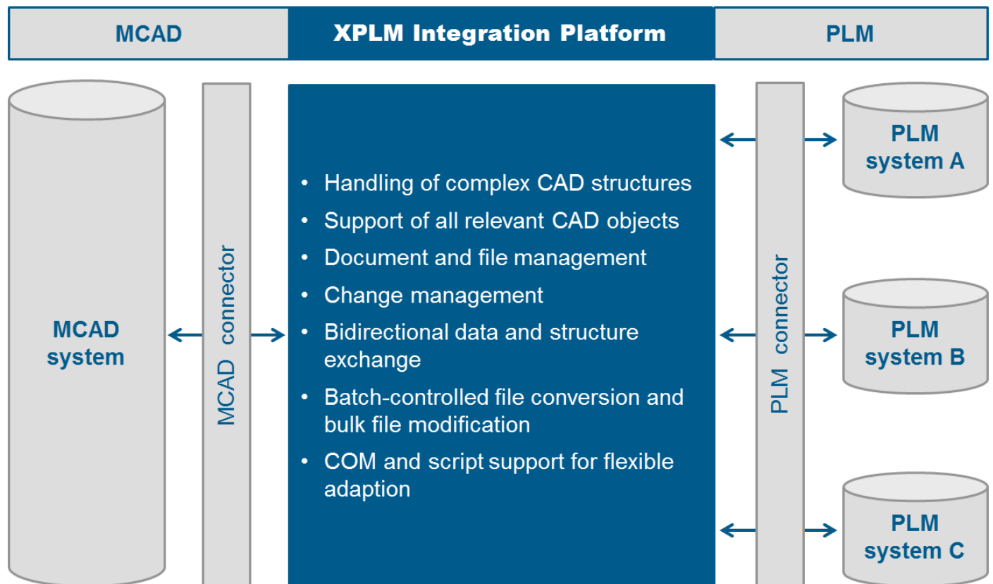
XPLM Integration Platform Datenfluss zwischen MCAD, PDM/PLM Systemen und ERP Systemen
